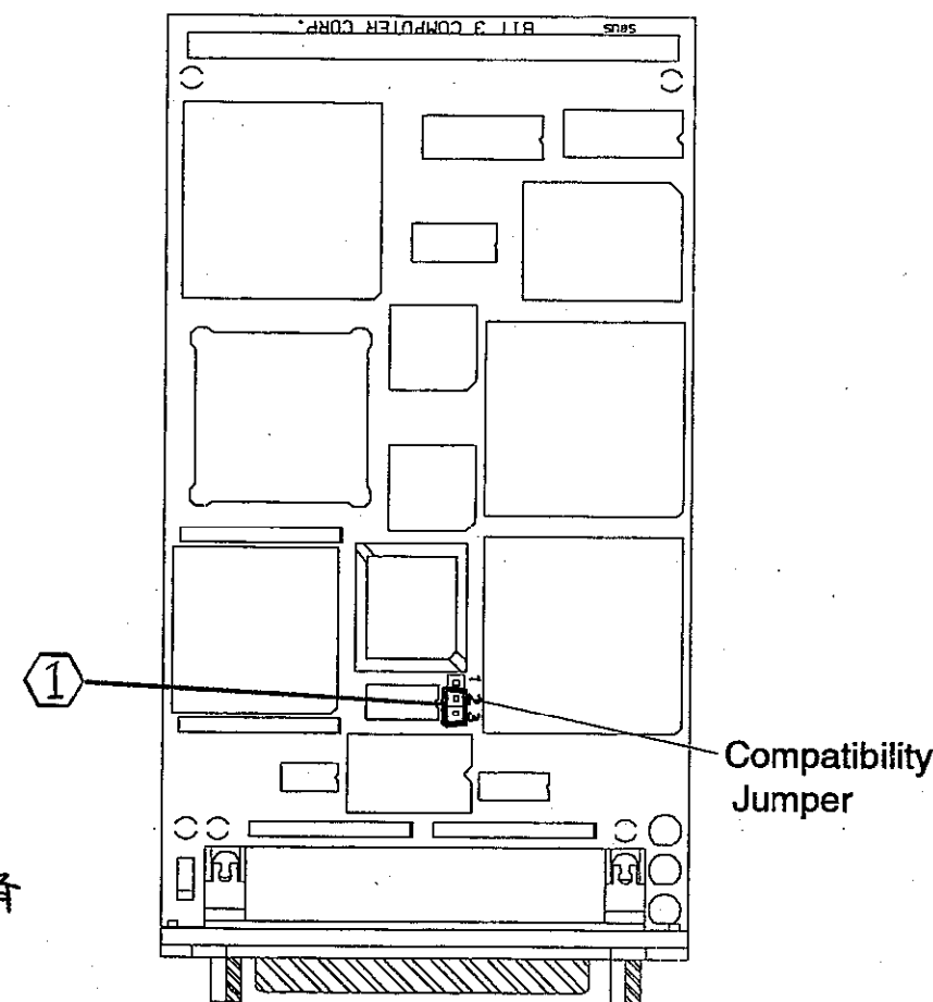
図2 Sバスカードの設定 △ (MODEL 467-1のみ設定する) JP setting for BIT3
